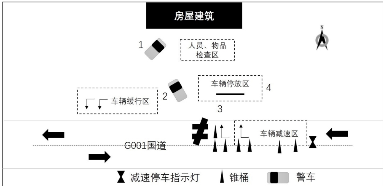
检查站示意图
